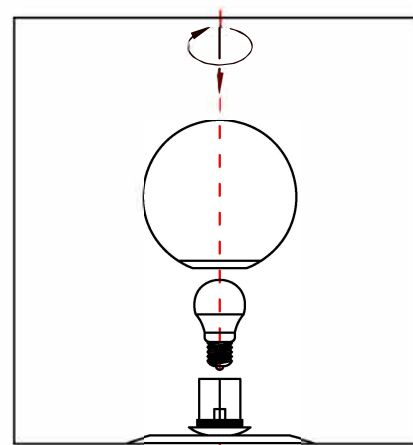
Schéma montáže stínidla. Installation diagram of lampshade.
