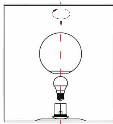
Schéma montáže stínidla.
